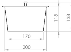
KARŞIDAN GÖRÜNÜM
